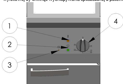
Rysunek 6 Panel sterowania
