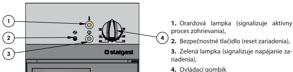
Obrázok 7 Ovládacie prvky zariadenia
