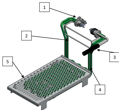
Obrázok 9. Ohrievacie teleso spolu s podstavcom pre košík
