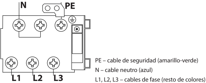
Figura 7. Conexión del equipo a la instalación eléctrica.
