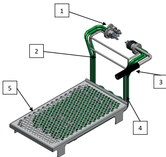
Figura 11. Calentador junto con la base de la cesta
