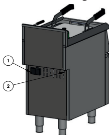
Fig. 4. Raccordement de l'appareil à une installation équipotentielle.
