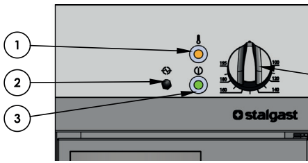
Figure 8 Composants du système de commande de l'appareil
