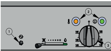
Figura 10. Elementos de control del dispositivo
