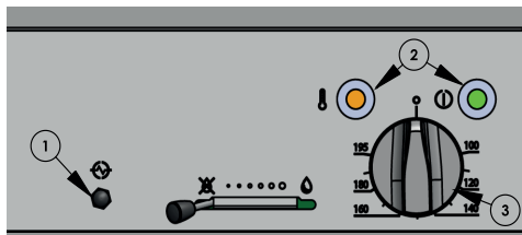
Obrázek č. 10. Řídící prvky přístroje
