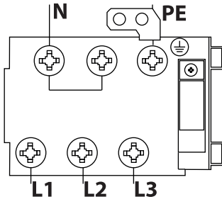
Figure 7. Branchement de l'appareil au réseau électrique.
