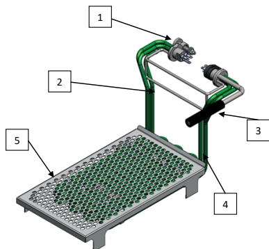
Bild 11 Heizelement mit der Korbunterlage
