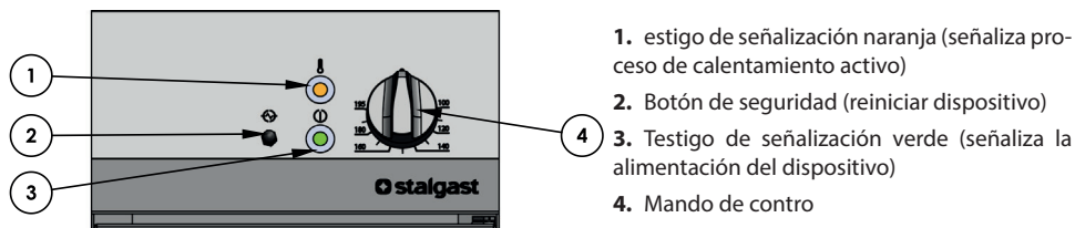
Figura 8. Elementos de control del dispositivo
