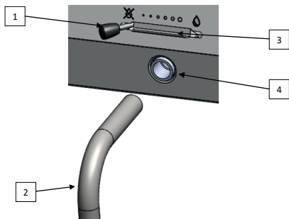
Obrázek č. 12. Prvky mechanismu pro vypouštění oleje
