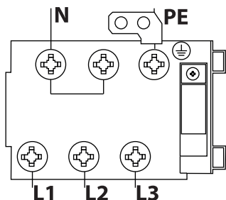
Obrázok 7. Pripojenie zariadenia do elektrickej siete
