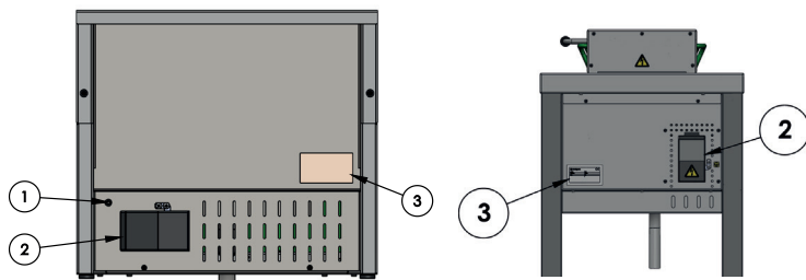
Obrázek č. 5. Náhled na přístroj 9725500 zezadu.
