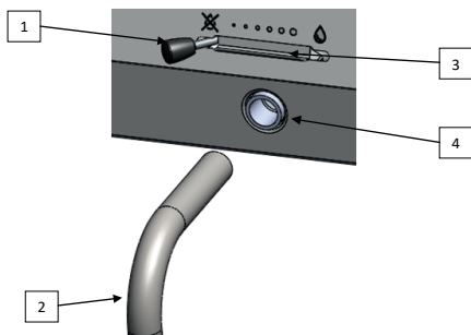
Obrázok 10. Prvky mechanizmu na vypúšťanie oleja
